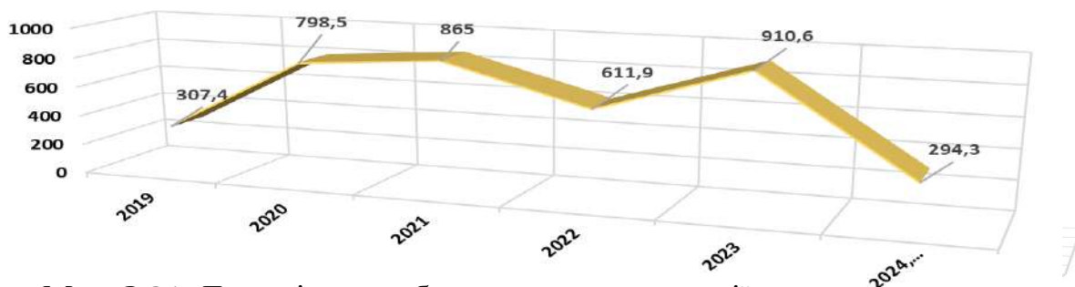
Мал. 3.21. Динаміка виробництва електроенергії сонячними електростанціями в Миколаївській області
